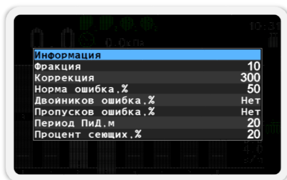
Рисунок 45 Параметры датчика высева
