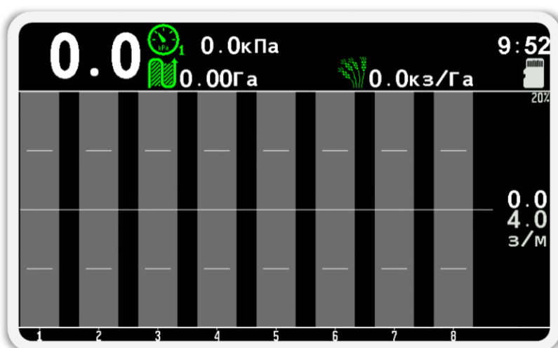
Рисунок 28 Пример отображения «Главного экрана» тогда, когда установлена связь со всеми датчиками и при этом все датчики поставлены на контроль.
