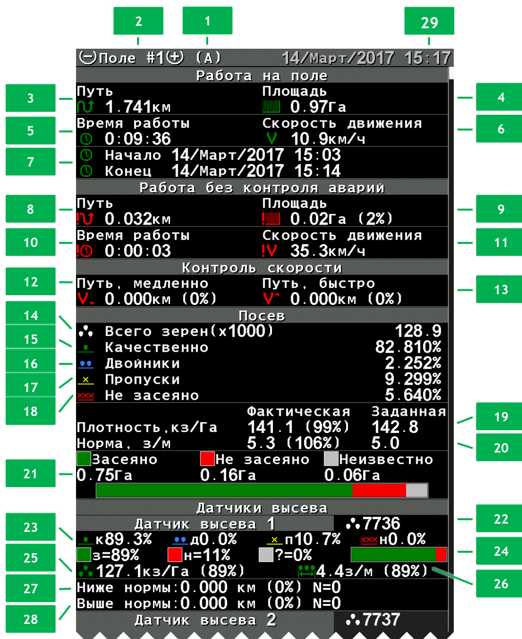
Рисунок 18 Содержимое статистики для режима контроля высева "Точный"
