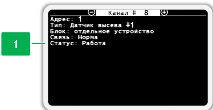
Рисунок 46 Экран просмотра состояния датчика контроля высева
