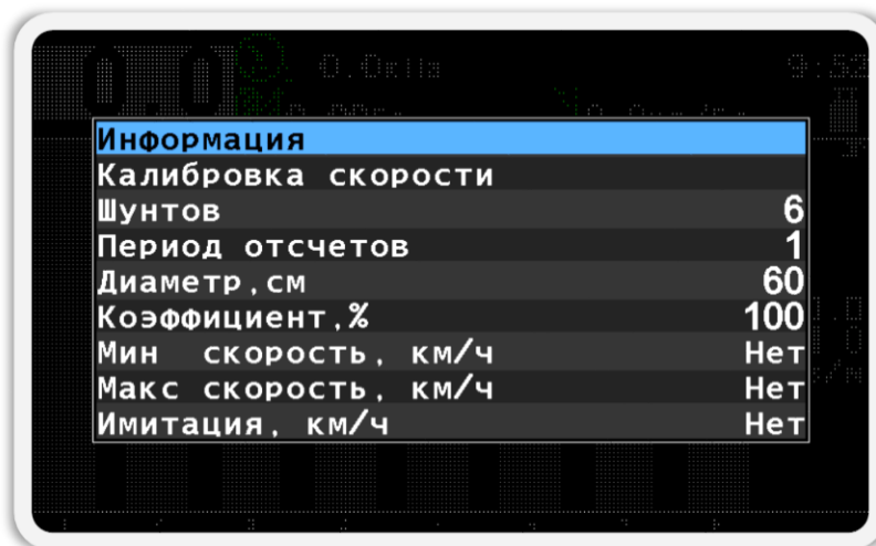
Рисунок 41 Параметры датчика скорости движения сеялки
