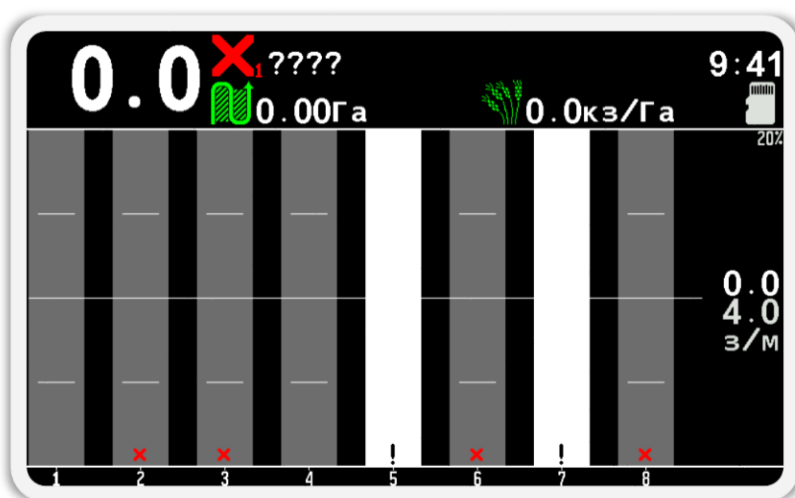
Рисунок 27 Пример отображения «Главного экрана» тогда, когда нет связи с некоторыми датчиками, а также некоторые датчики сняты с контроля.
