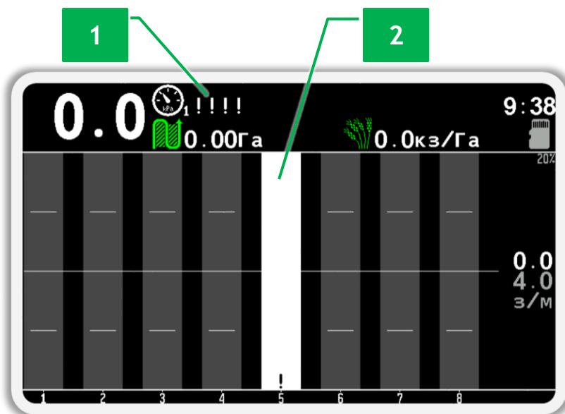
Рисунок 23 Пример отображения снятых с контроля датчиков. Сняты с контроля следующие датчики: 1 - датчик давления; 2 - датчик контроля высева №5.
